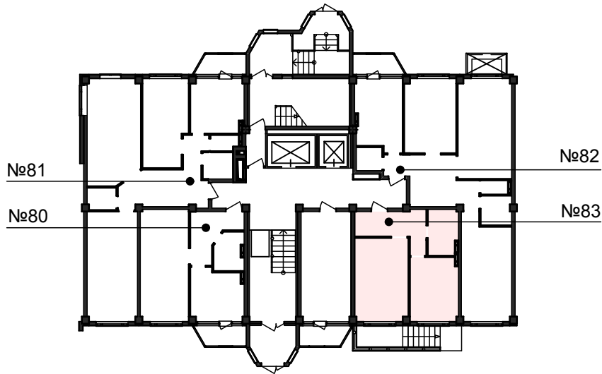
СХЕМА СЕКЦИИ №2 (1 этаж)
