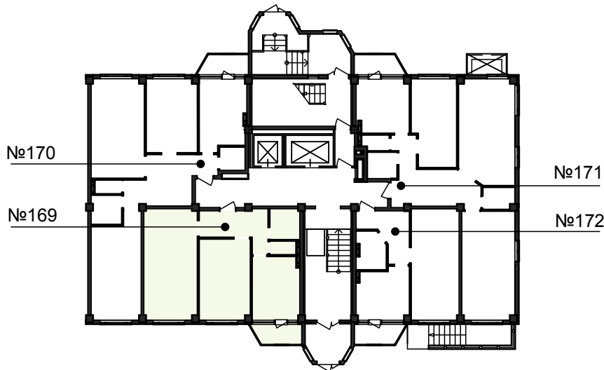
СХЕМА СЕКЦИИ №4 (1 этаж)
