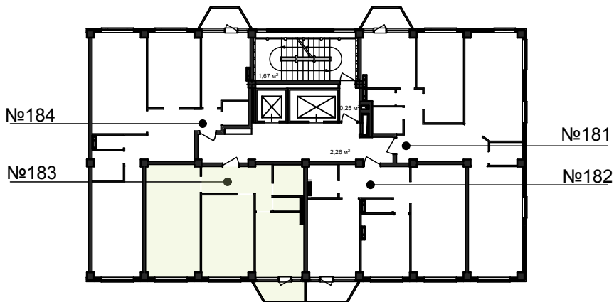
СХЕМА СЕКЦИИ №4 (4 этаж)
